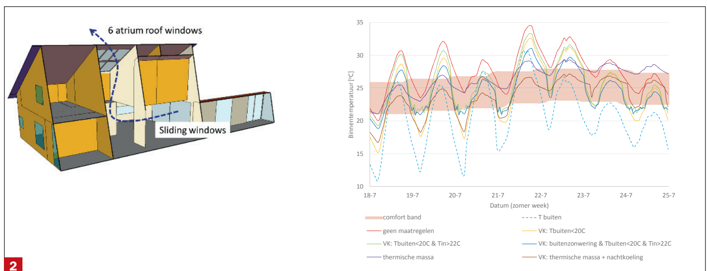
Gesimuleerde binnentemperaturen voor een zomerweek bij toepassing van verschillende controle en ontwerpstrategieën (VK: strategie die gebruik maakt van vrije koeling). 'Comfort band' geeft de comfort bandbreedte aan voor de bijbehorende buitencondities. 'T buiten ' is de buitentemperatuur, 'T in ' de binnentemperatuur. Figuren uit [9]
