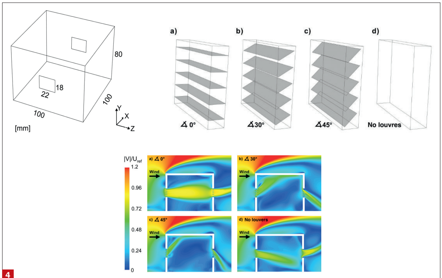
Contourplots van de dimensieloze snelheid ( |V|/U_{ref} ) in het verticale vlak van een eenvoudige geometrie voor een niet-isotherme simulatie bij verschillende hoeken van de louvers: (a) 0°, (b) 30°, (c) 45°, en voor (d) raam zonder louvers. U_{ref} = 6.97 m/s. Figuren uit [15]
