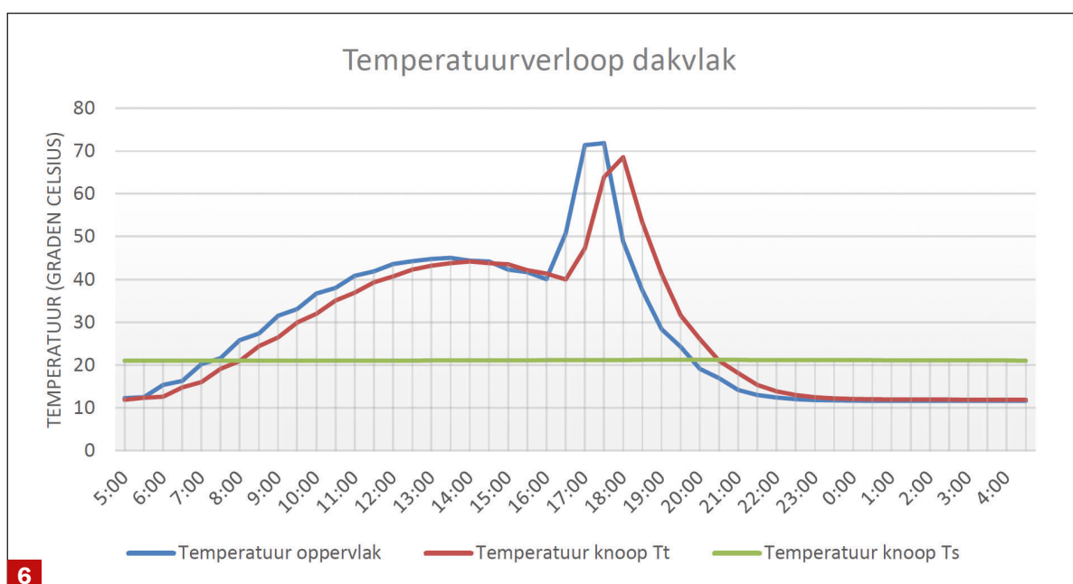
Zichtbare sprong in oppervlaktetemperatuur van een dak bij het optreden van een brandpunt op dat dakvlak [8]
