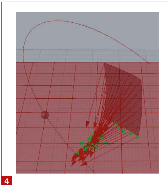
Van enkel- naar dubbelgekromd vlak, met reflecties en brandpunt [6]
