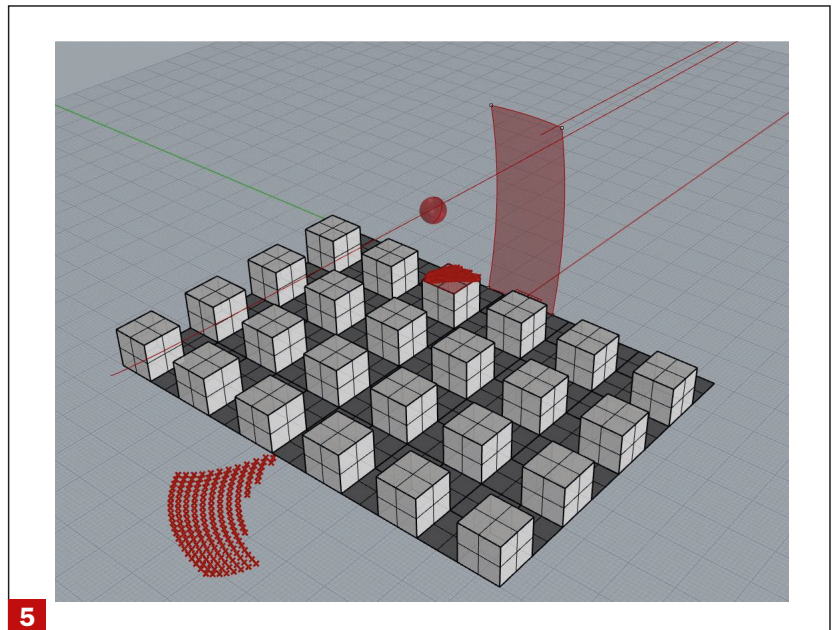
Brandpunt dat ontstaat op een dakvlak op 29 juli [8]
