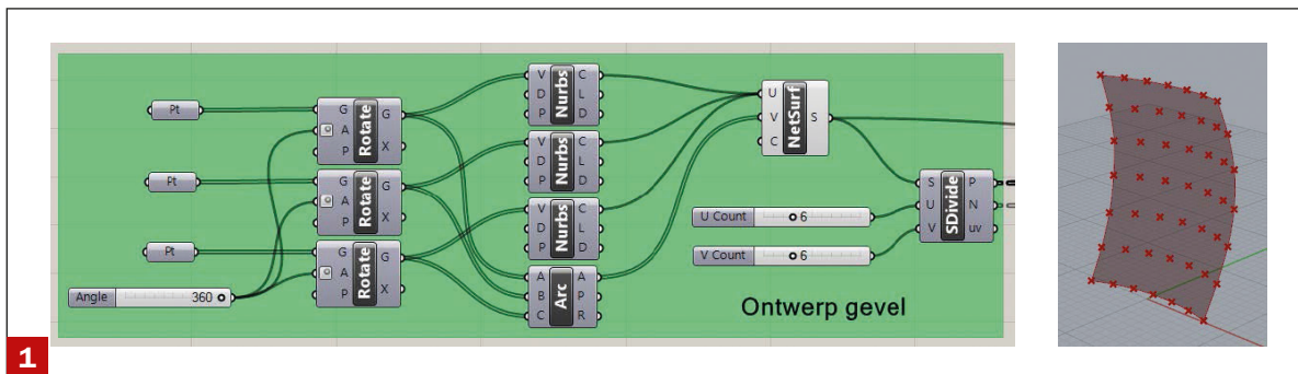
Voorbeeld associatief-geometrisch model in Grasshopper (links) met als resultaat dubbelgekromd geveloppervlak met verdeling in meetpunten (rechts) [6]
